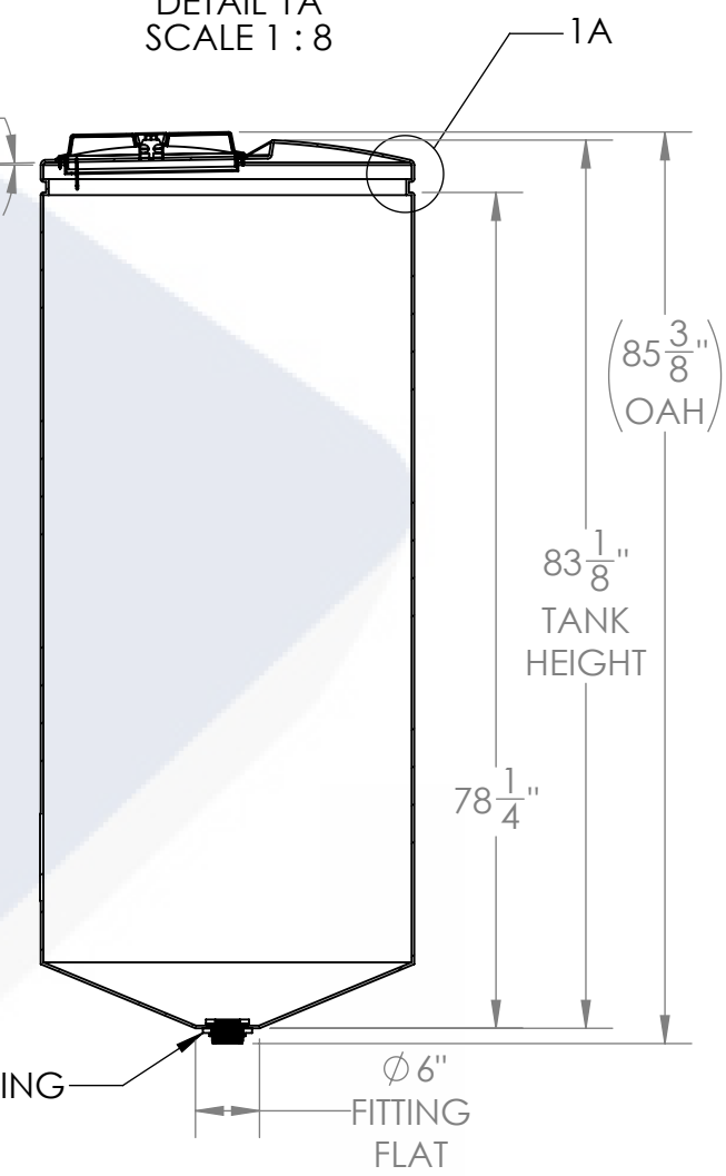
SECTION 1B-1B
